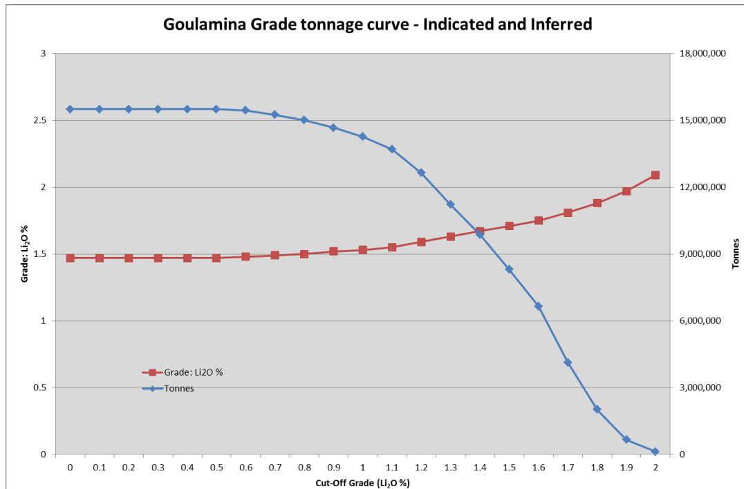
Abbildung 5. Goulamina Gehalt-Tonnage-Kurve.
