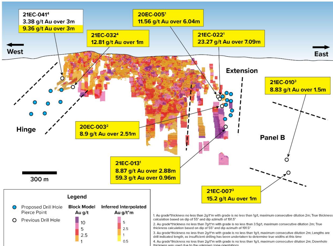
Abbildung 1: Längsschnitt der Lagerstätte Eau Claire mit ausgewählten Bohrhighlights aus dem Jahr 2021 sowie den Ansatzpunkten für die im Jahr 2022 geplanten Bohrungen.
