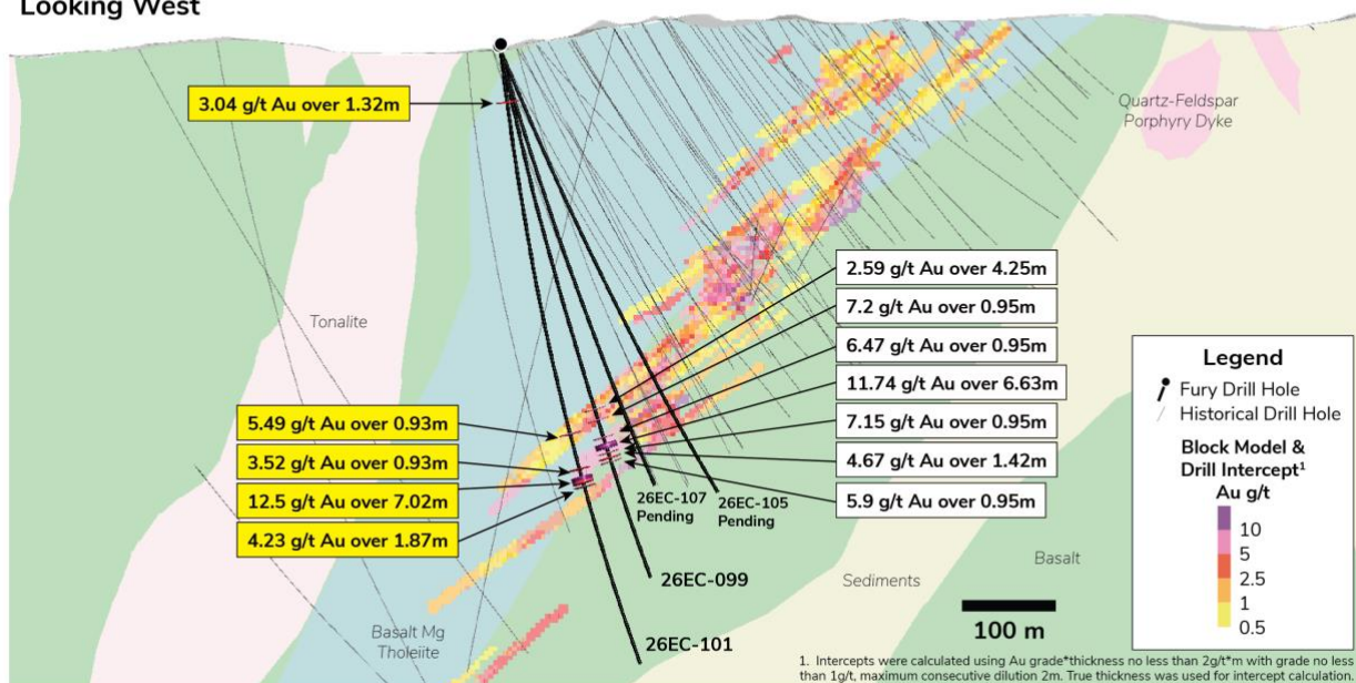
Abbildung 3: Eau Claire – Schnitt der Bohrlöcher 26EC-099 und 26EC-101
