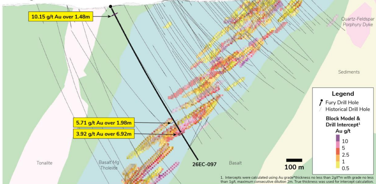
Abbildung 4: Eau Claire – Schnitt 26EC-097
