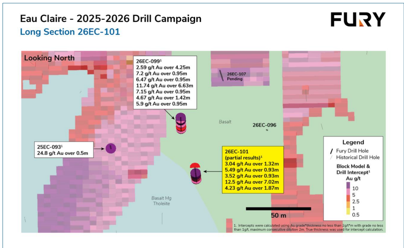
Abbildung 2: Eau Claire – Längsschnitt 26EC-101
