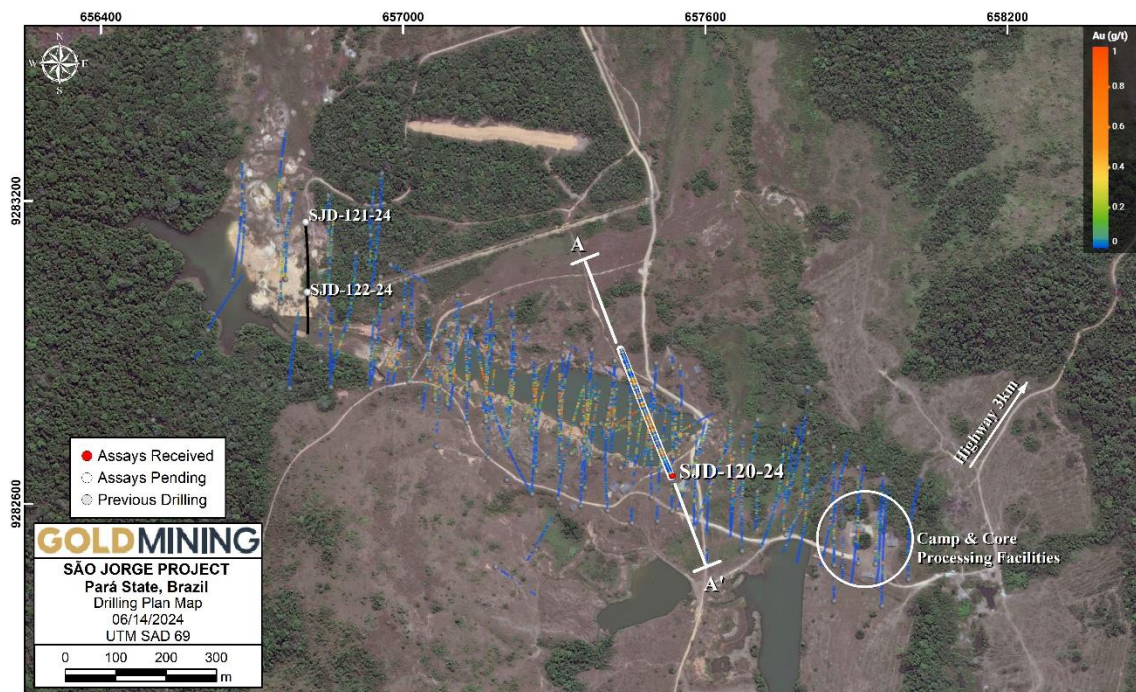
Abbildung 2 - Standorte der Bohrlöcher der Goldlagerstätte São Jorge, einschließlich des Standorts von SJD-120-24 und anderer Bohrlöcher, deren Untersuchungsergebnisse noch ausstehen. Die in Abbildung 3 dargestellte Schnittlinie ist eingezeichnet.
