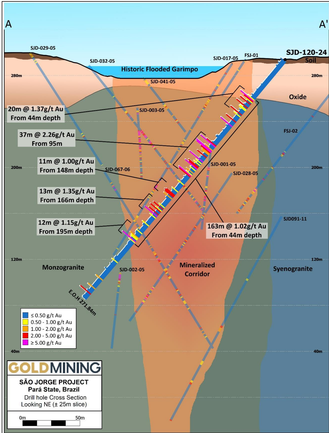
Abbildung 3 - Querschnitt der Bohrlöcher der Goldlagerstätte São Jorge, der den Standort des vor kurzem abgeschlossenen Bohrlochs SJD-120-24 zeigt und nach Nordosten ausgerichtet ist (siehe Schnittzeichnung in Abbildung 2).
