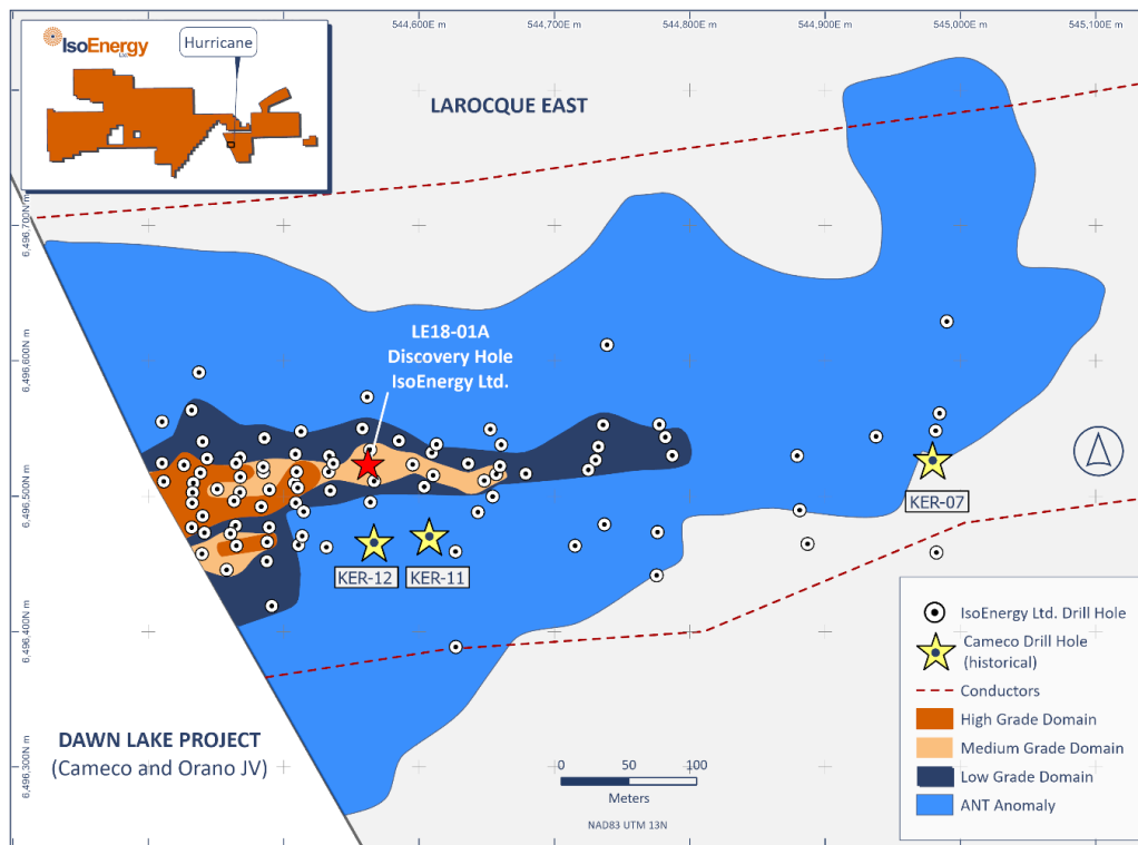
Abbildung 2 - Der Grundriss der Lagerstätte Hurricane, der die unmittelbare Nähe der drei Vorentdeckungsbohrlöcher (KER-07, 11 & 12) und des Entdeckungsbohrlochs LE18-01A von IsoEnergy
