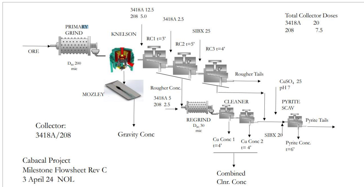
Abbildung 3: Das für die PFS entwickelte RevC-Prozessfließdiagramm
