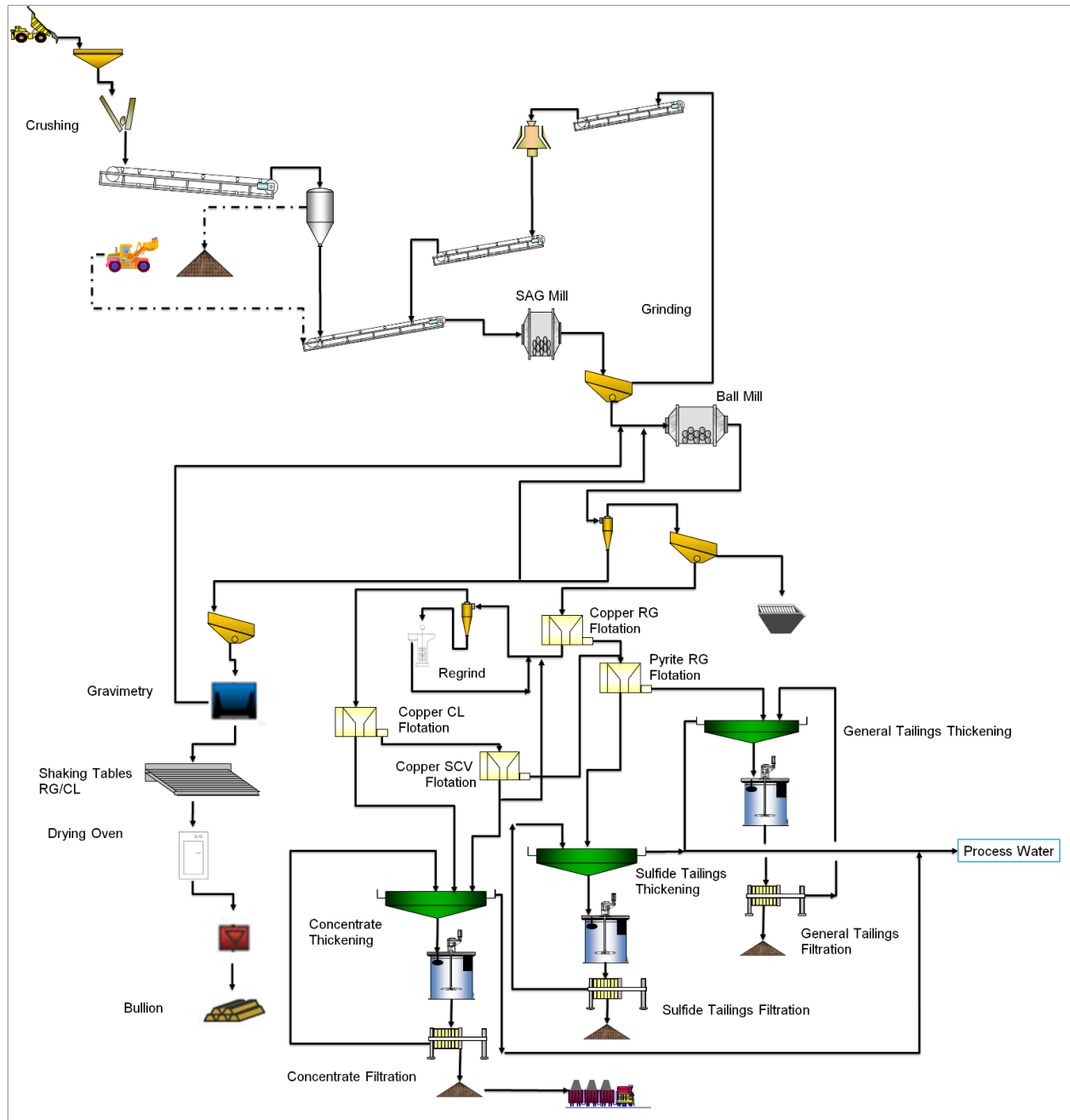
Abbildung 5: Aufbau der Prozessanlage Cabaçal
