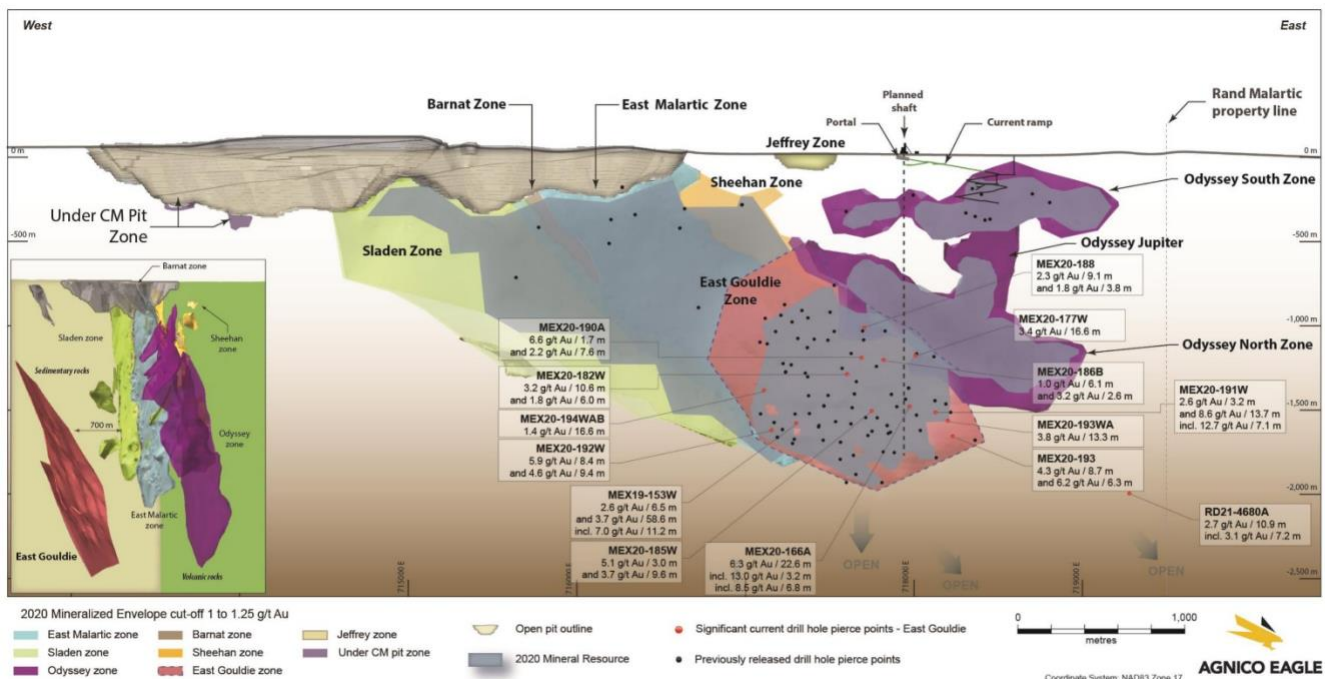
Abbildung 1. Zusammengesetzter Längsschnitt aus der Pressemitteilung von Agnico Eagle vom 29. April 2021 mit Explorationshighlights auf der Lagerstätte East Gouldie.
