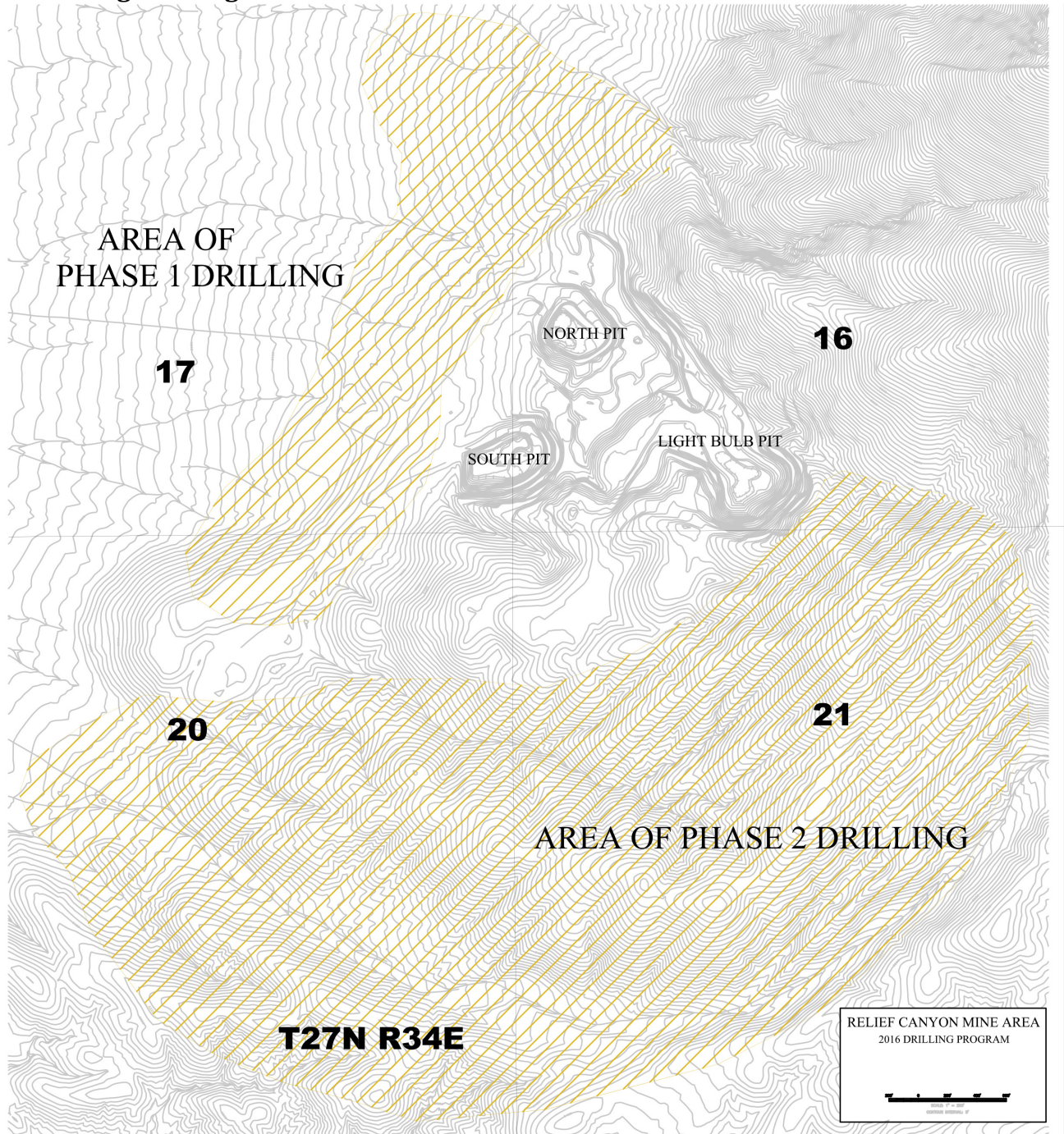
Abbildung 1: Bohrgebiete der Phase 1 und Phase 2
