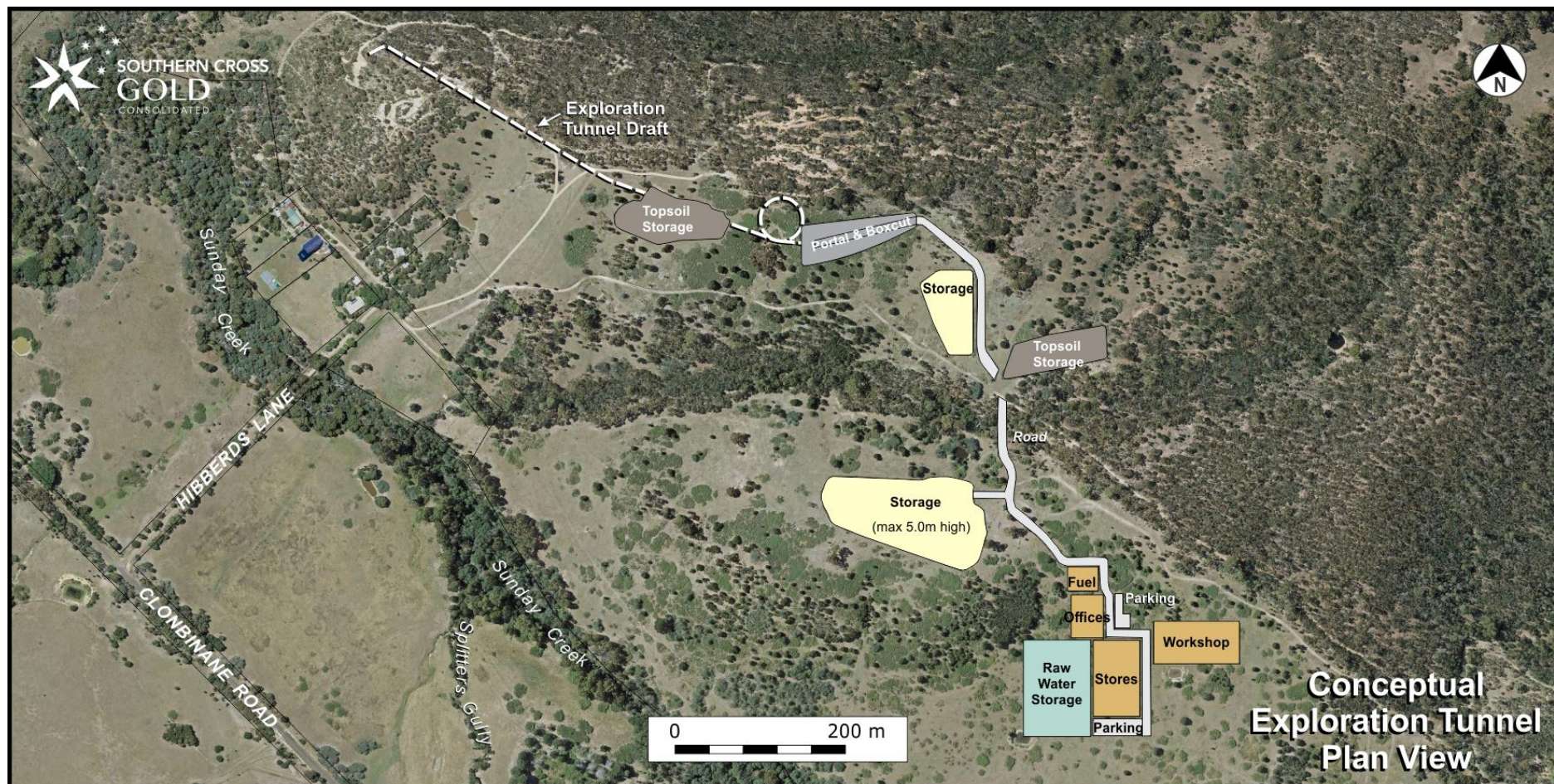
Abbildung 1: Draufsicht auf Sunday Creek mit konzeptioneller Darstellung der Oberfläche und des unterirdischen Tunnelverlaufs.
