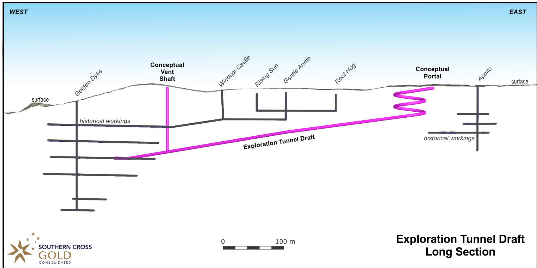
Abbildung 2: Längsschnitt des Explorationstunnels in Sunday Creek.
