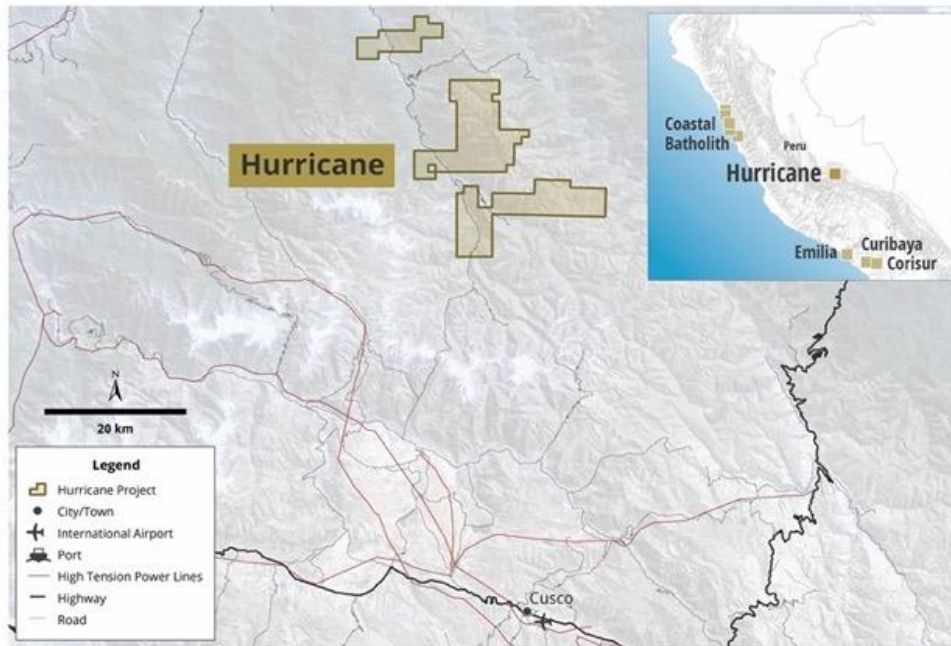
Abbildung 1: Zeigt die Lage des Hurricane-Projekts im Südosten Perus, etwa 60 km nördlich von Cusco.
