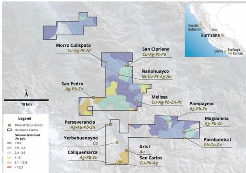
Abbildung 4: Veranschaulicht anomales Gold in Entwässerungsbecken auf den bekannten Schürfstellen.
