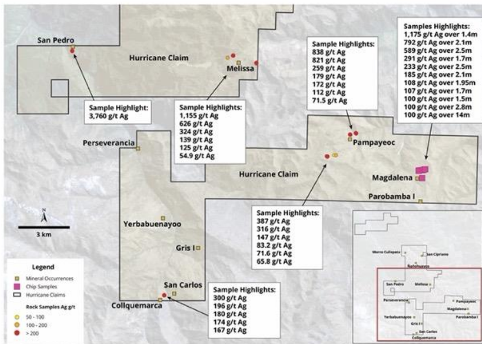
Abbildung 2: Veranschaulicht die Höhepunkte der Silbergehalte von Gesteinsschürfproben aus mehreren Schürfbereichen innerhalb des Projektgebiets Hurricane.
