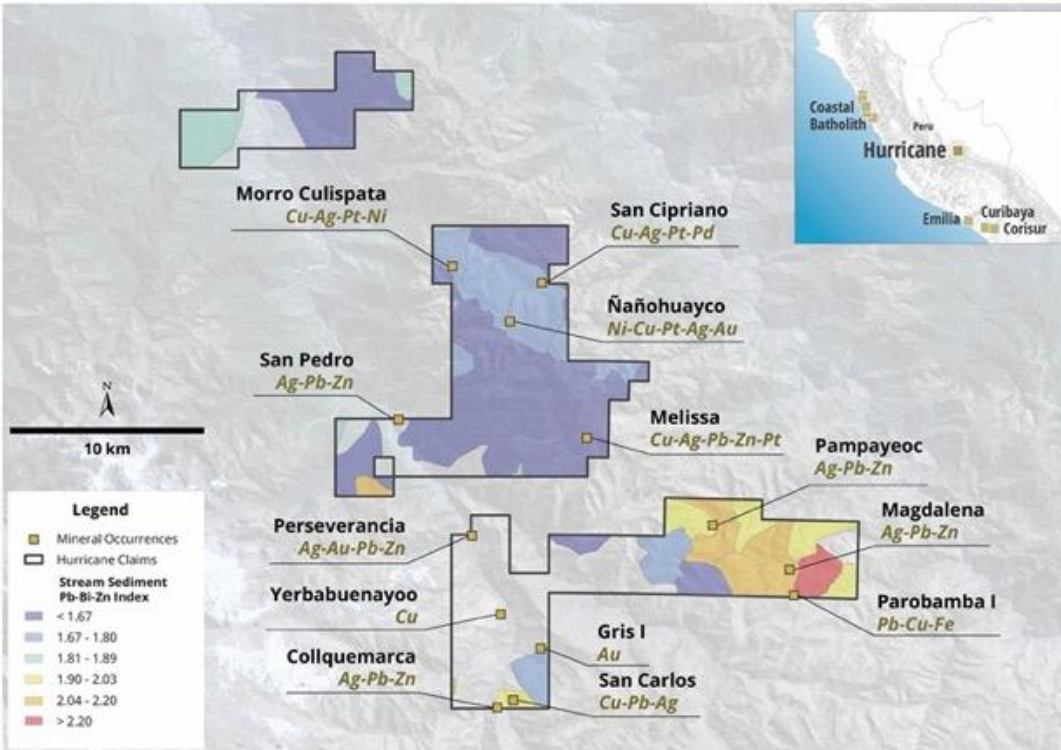
Abbildung 6: Veranschaulicht Blei-Wismut-Zink-Anomalien in Entwässerungsbecken, von denen man annimmt, dass sie mit Mineralisierungsarten mit mittlerer Sulfidierung in Verbindung stehen.
