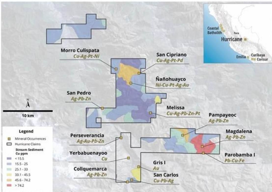
Abbildung 5: Veranschaulicht anomales Kupfer in Entwässerungsbecken in den bekannten Schürfgebieten.
