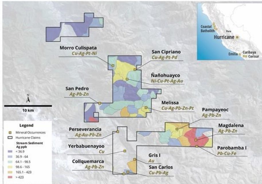
Abbildung 3: Veranschaulicht anomales Silber in Entwässerungsbecken auf den bekannten Schürfstellen.
