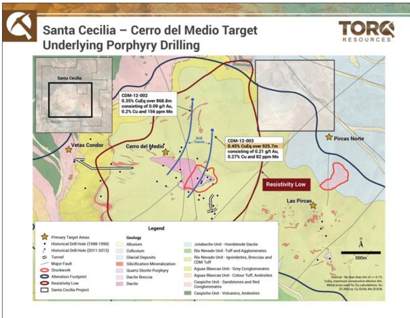
Abbildung 2: Veranschaulicht das Zwei-Loch-Bohrprogramm, das von Januar 2012 bis Mai 2012 durchgeführt wurde, um die Porphyrymineralisierung unterhalb der oberflächlichen epithermalen Mineralisierung zu erproben, die bei den Bohrungen des vorherigen Betreibers entdeckt wurde. Die beiden Bohrlöcher wurden von der Nordseite der topografischen Erhebung aus gebohrt, die das Zielgebiet Cerro del Medio definiert, und beide durchschnitten Hunderte von Metern mit einer Gold-Kupfer-Molybdän-Mineralisierung im Porphyry-Stil.
