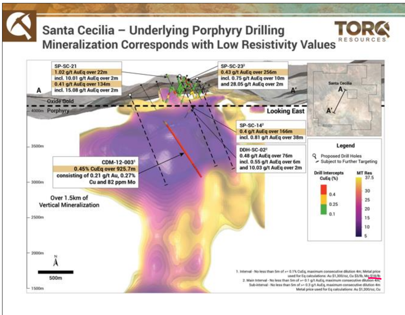
Abbildung 3: Zeigt eines der beiden Bohrlöcher, die 2012 gebohrt wurden, um eine Porphyrymineralisierung unterhalb der epithermalen Mineralisierung zu finden, die bei den Bohrungen des vorherigen Betreibers entdeckt wurde. Wichtig ist, dass die Gold-Kupfer-Porphyr-Mineralisierung einem 2 km x 2 km x 1 km großen Gebiet mit niedrigen Widerstandswerten entspricht, das sowohl in geophysikalischen Untersuchungen mit induzierter Polarisierung als auch mit magneto-tellurischen Messungen definiert wurde, wobei die Mineralisierung in der Tiefe und seitlich offen ist.
