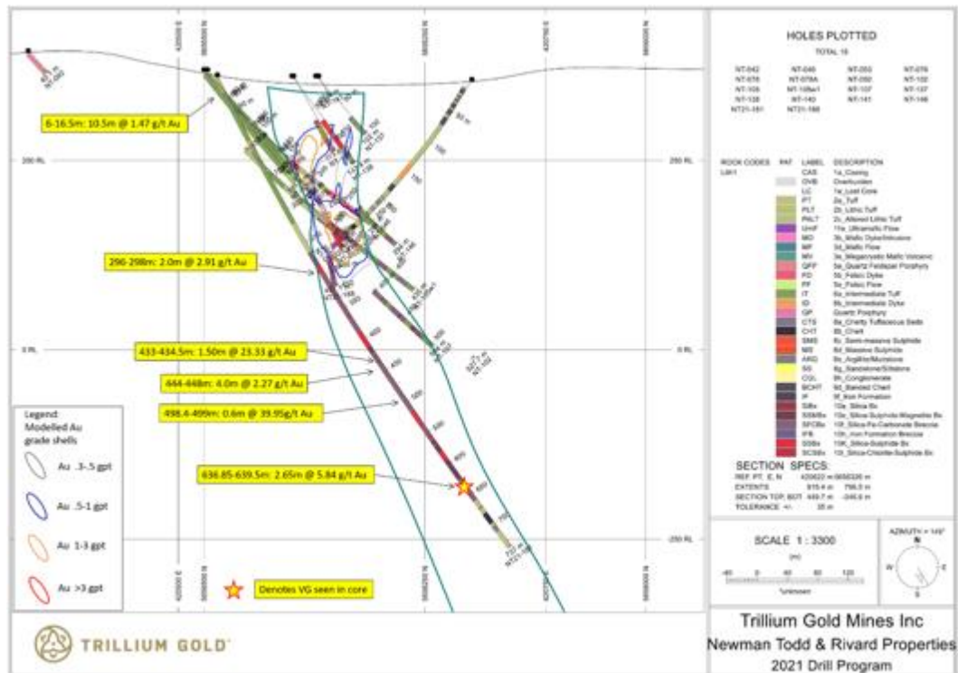
Abbildung 3: Schnitt für das Bohrloch NT21-181 mit signifikanten mineralisierten Abschnitten.
