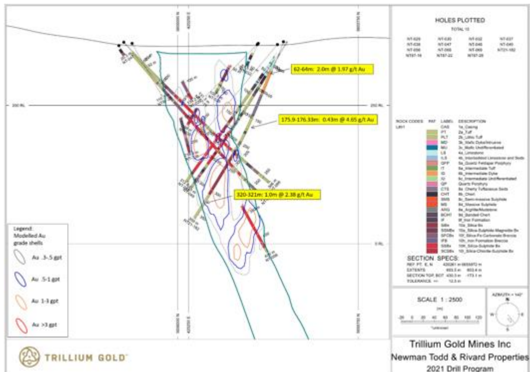
Abbildung 4: Schnitt für Bohrloch NT21-182 mit signifikanten mineralisierten Abschnitten.
