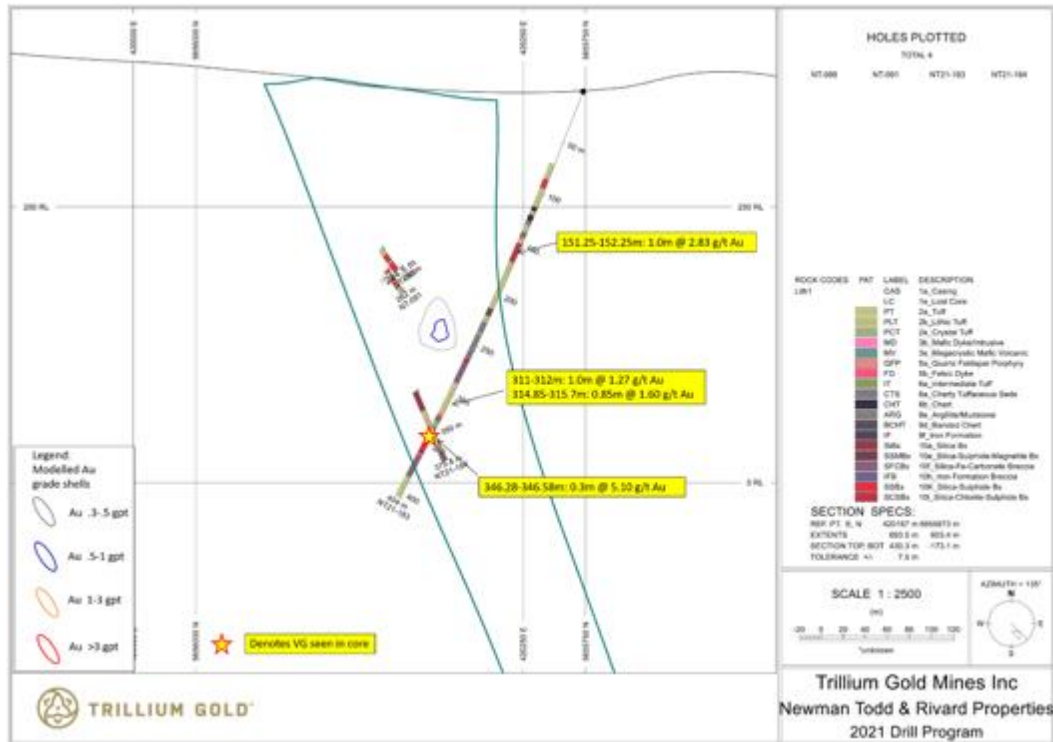
Abbildung 5: Schnitt für Bohrloch NT21-183 mit signifikanten mineralisierten Abschnitten.
