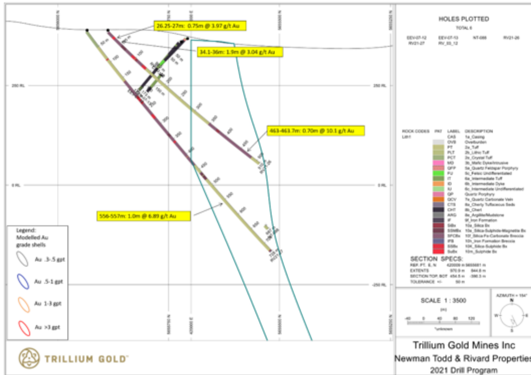
Abbildung 7: Schnitt durch die Bohrlöcher RV21-26 & RV21-27 mit signifikanten mineralisierten Abschnitten.
