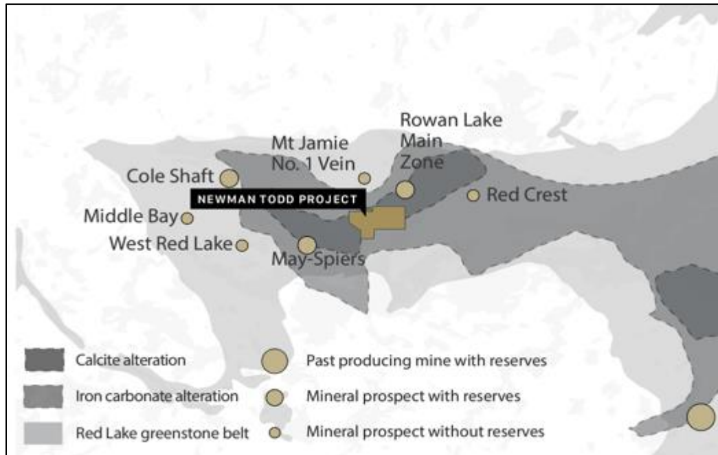
Abbildung 2: Lage des Projekts Newman Todd, das sich nun zu 100 % im Besitz von Trillium Gold Mines befindet, einschließlich der produzierenden und ehemals produzierenden Minen, der Mineralprospekte sowie des Red Lake Greenstone-Gürtels, der Geologie und der Alterationspakete
