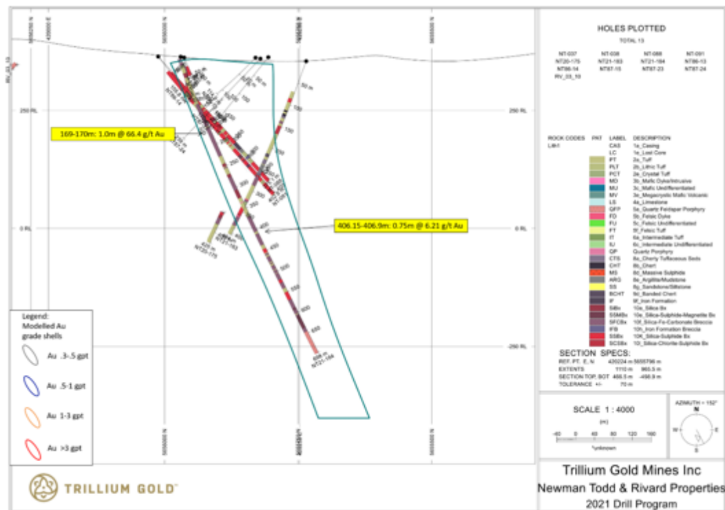
Abbildung 6: Schnitt für Bohrloch NT21-184 mit signifikanten mineralisierten Abschnitten.
