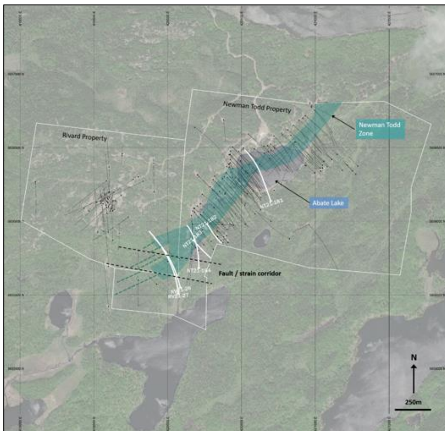
Abbildung 1: Draufsicht auf die Grundstücke Newman Todd / Rivard, die Zone NT und die 6 Bohrlöcher, über die in dieser Pressemitteilung berichtet wird.
