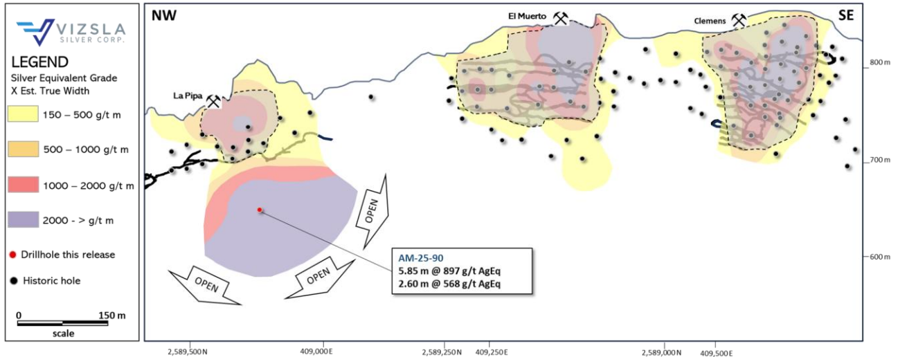
Abbildung 2: Längsschnitt der Animas-Struktur mit historischen Bohrlochdurchstichen (schwarz) und Bohrloch AM-25-90 (rot), das eine hochgradige Mineralisierung unterhalb der historischen Minenanlagen bei La Pipa erschließt. Die grauen Polygone mit der schwarzen gestrichelten Linie stellen die geschätzte hochgradige Mineralisierung dar, die von lokalen Bergleuten auf den oberen 100 Metern der Ader abgebaut wurde.
