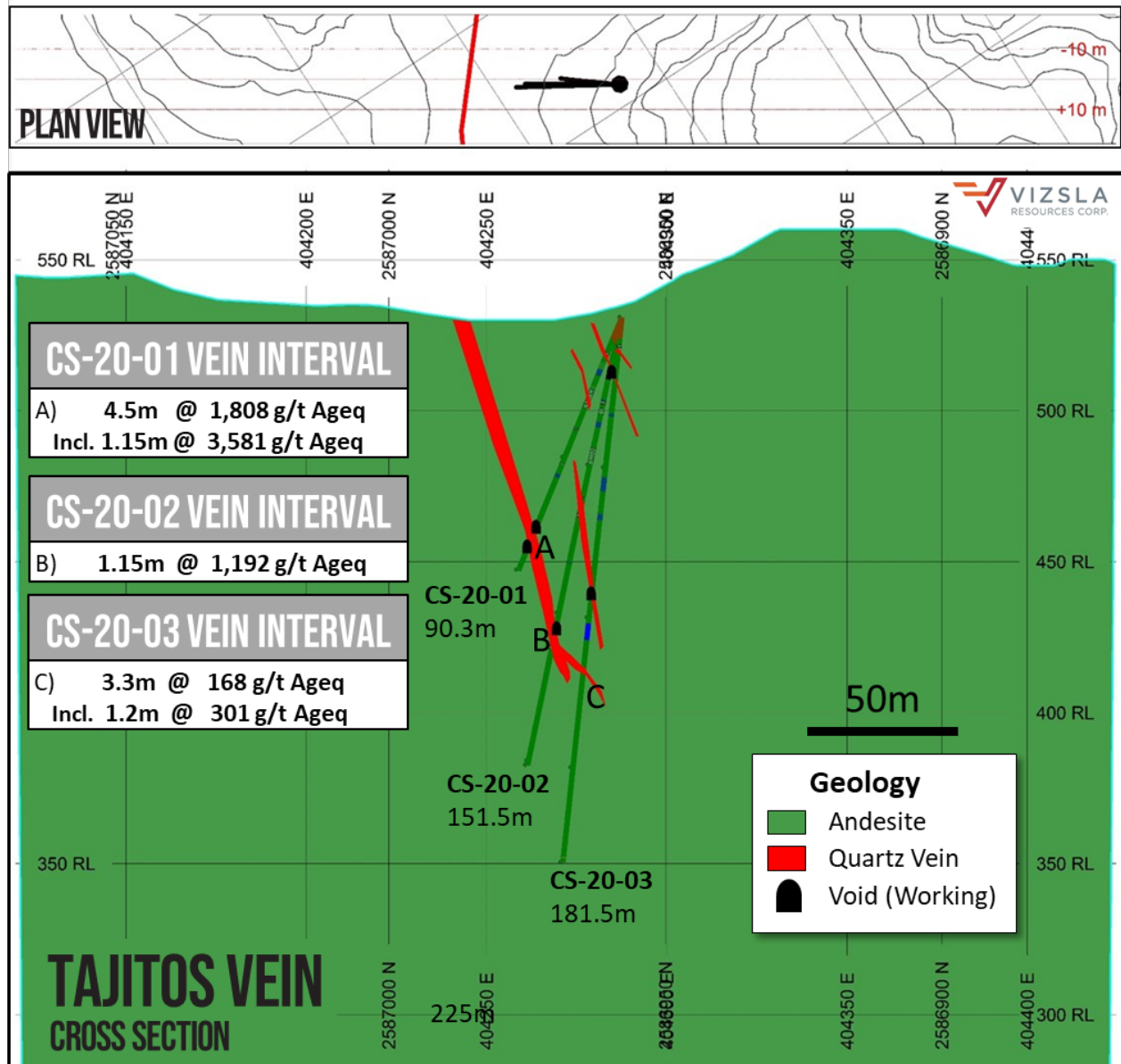
Abbildung 3: Profilschnitt durch Bohrungen CS-20-01, CS-20-02 und CS-20-03, Erzgang Tajitos.
