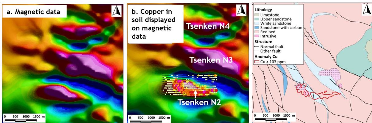
Abbildung 1. Das Ziel von Tsenken N2: a. Reduzierung auf die Polverarbeitung ("RTP") von aeromagnetischen Daten im Bereich des Tsenken Nord. Violette und rote Farben stellen stark
