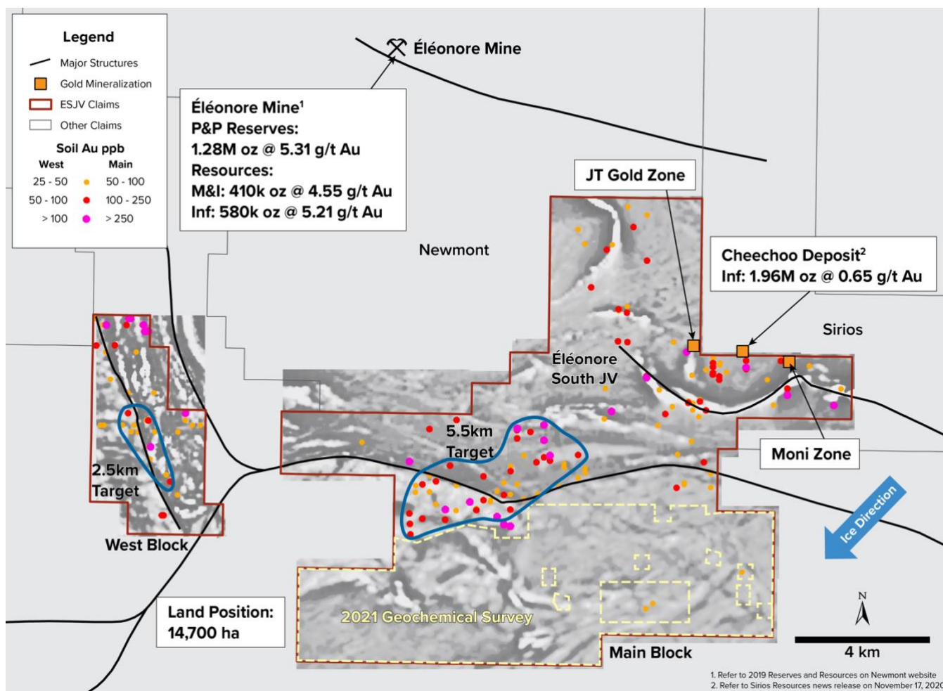
Abbildung 2: Veranschaulicht die beiden großflächigen geochemischen Anomalien, die die beiden Zielgebiete darstellen, die die Fury im Jahr 2021 bis zum Bohrstadium vorantreiben möchte, sowie den Standort der erweiterten geochemischen Untersuchung im südlichen Drittel des Grundstücks.
