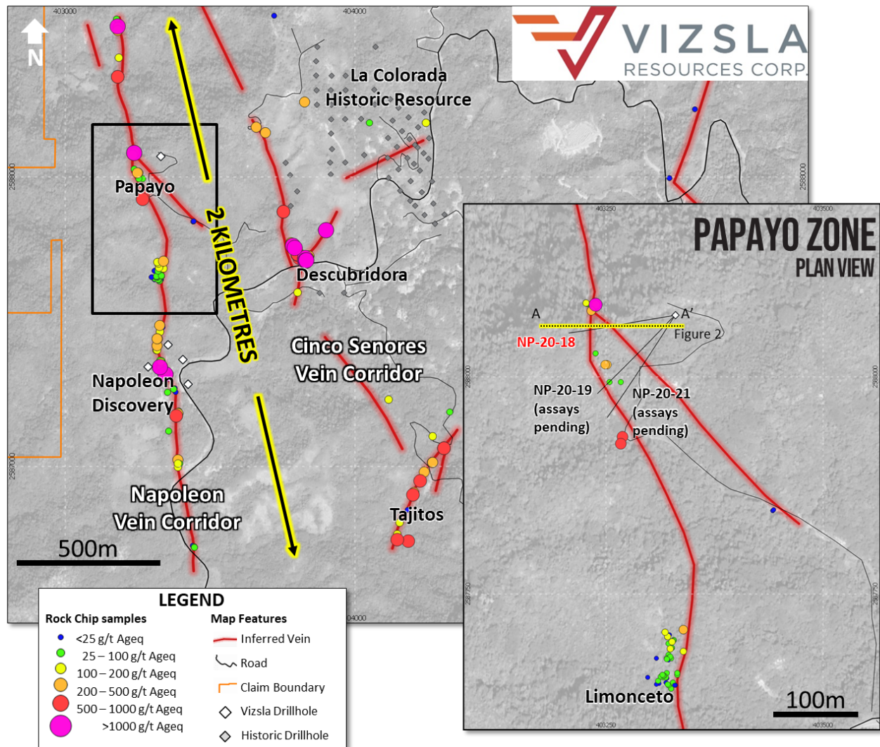
Abbildung 1: Karte mit Lage der Bohrungen, kartierten Erzgängen sowie Übertage- und Untertageprobenentnahmen im Prospektionsgebiet Papayo auf dem Gangsystem Napoleon. Nebenkarte zeigt Details der Bohransatzpunkte.
