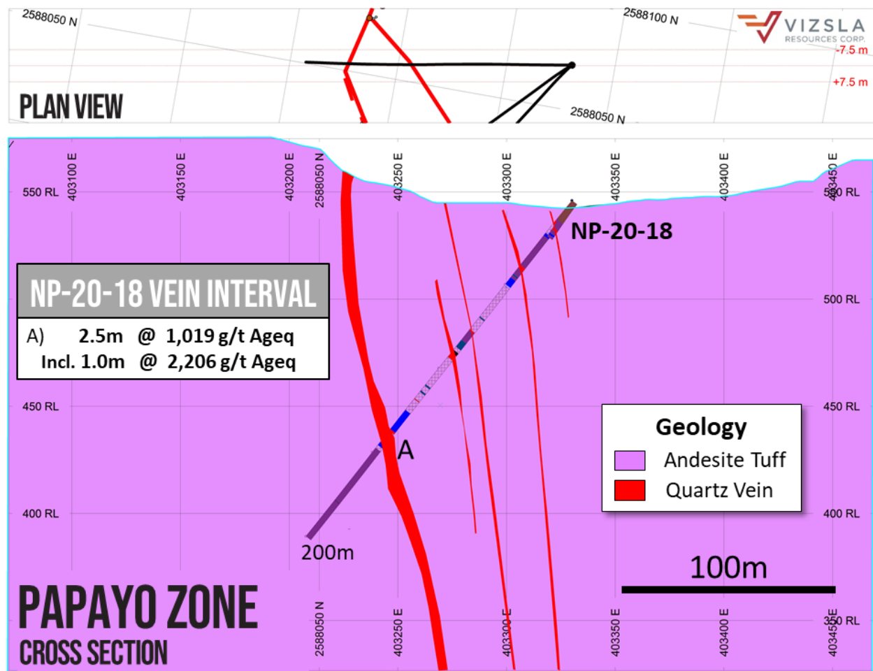
Abbildung 2: Profilschnitt durch Bohrung NP-20-18.
